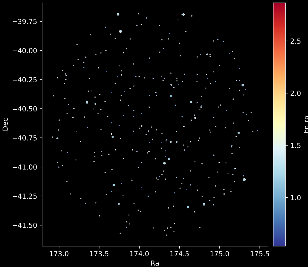
GALAH DR4 Field: [337] Stars: 300
