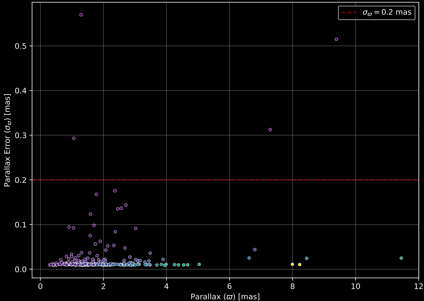
GALAH DR4 Field: [337] Parallax Quality (n= 300)
