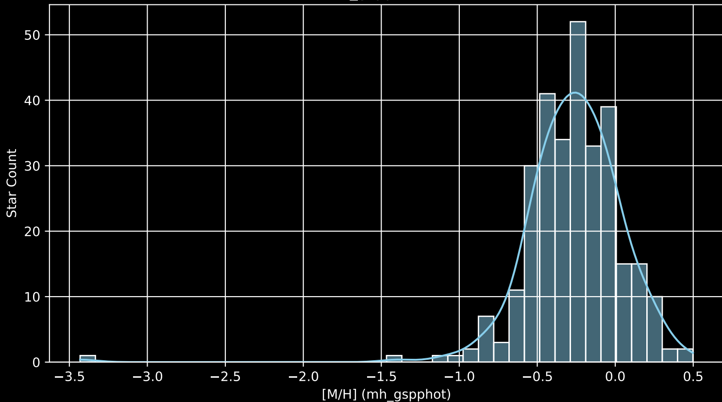
GALAH DR4 Field: [337] [M/H] (mh_gspphot) (n= 300)
